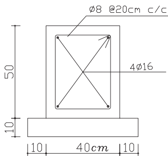
مقطع شناژ
